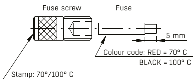
Fig. 1. Fuse
