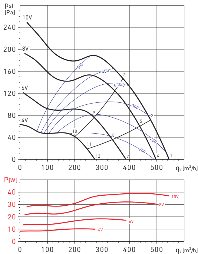
TD-500/150-160 SILENT ECOWATT
